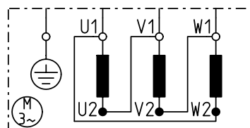
Dreieckschaltung
