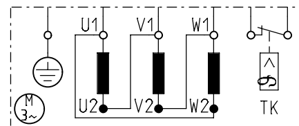
Dreieckschaltung/delta wiring
